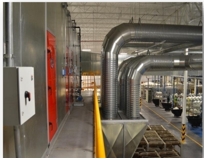
Red de ductos para colección de fibras y polvos
